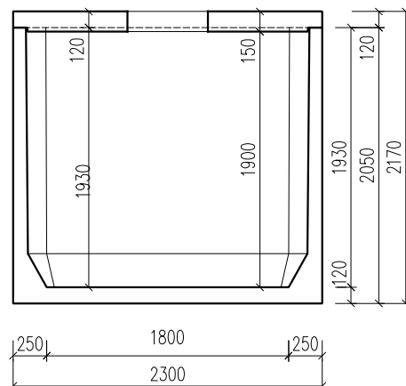
ŘEZ B-B
