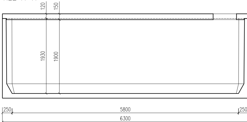
ŘEZ A-A
