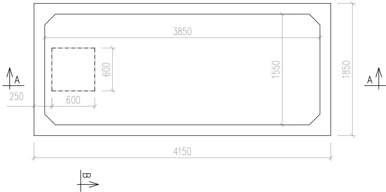
PŮDORYS
