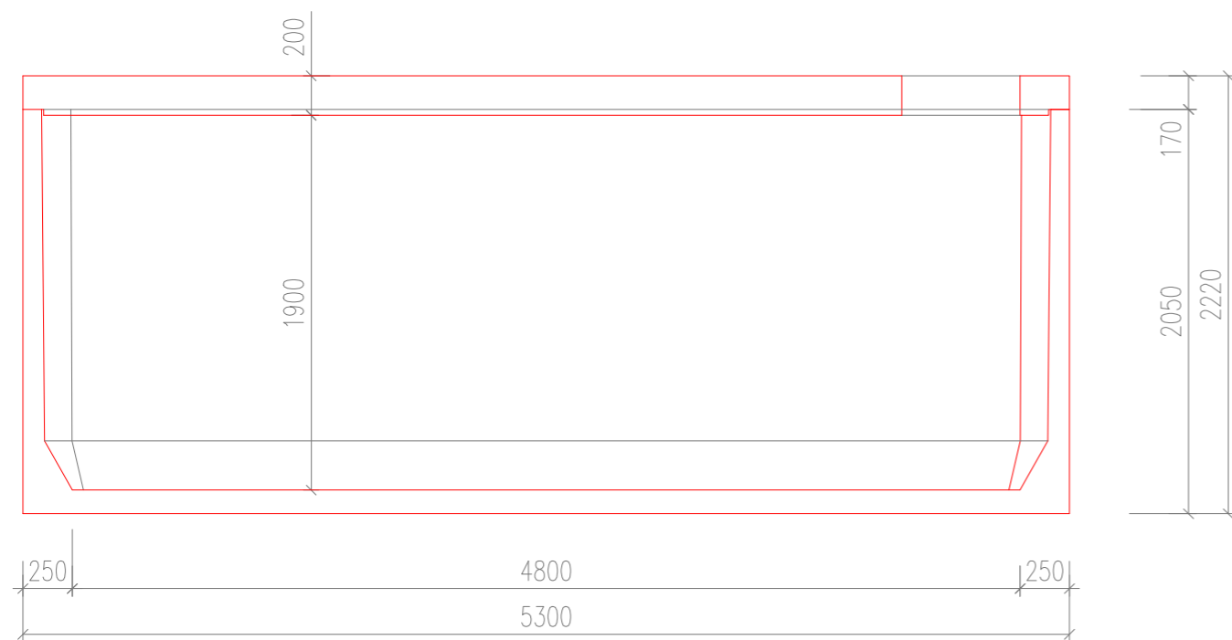
ŘEZ A-A'
