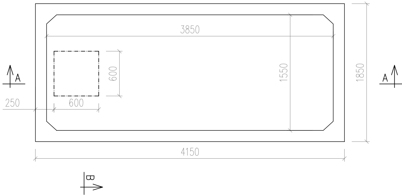
PŮDORYS
