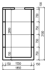
ŘEZ B-B'
