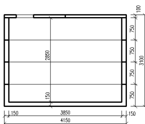
ŘEZ B-B'
