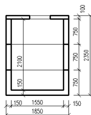
ŘEZ B-B'
