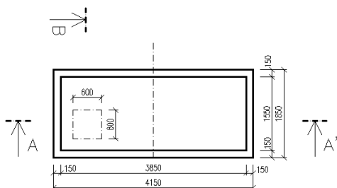
PŮDORYS:
