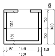
ŘEZ B-B'
