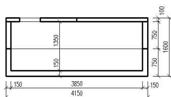
ŘEZ B-B'
